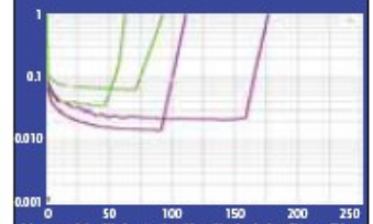
Unterschiedlich starke Kanäle bei der Eton. Die grünen Klirrverläufe gehören zu den Kanälen 1 und 2
